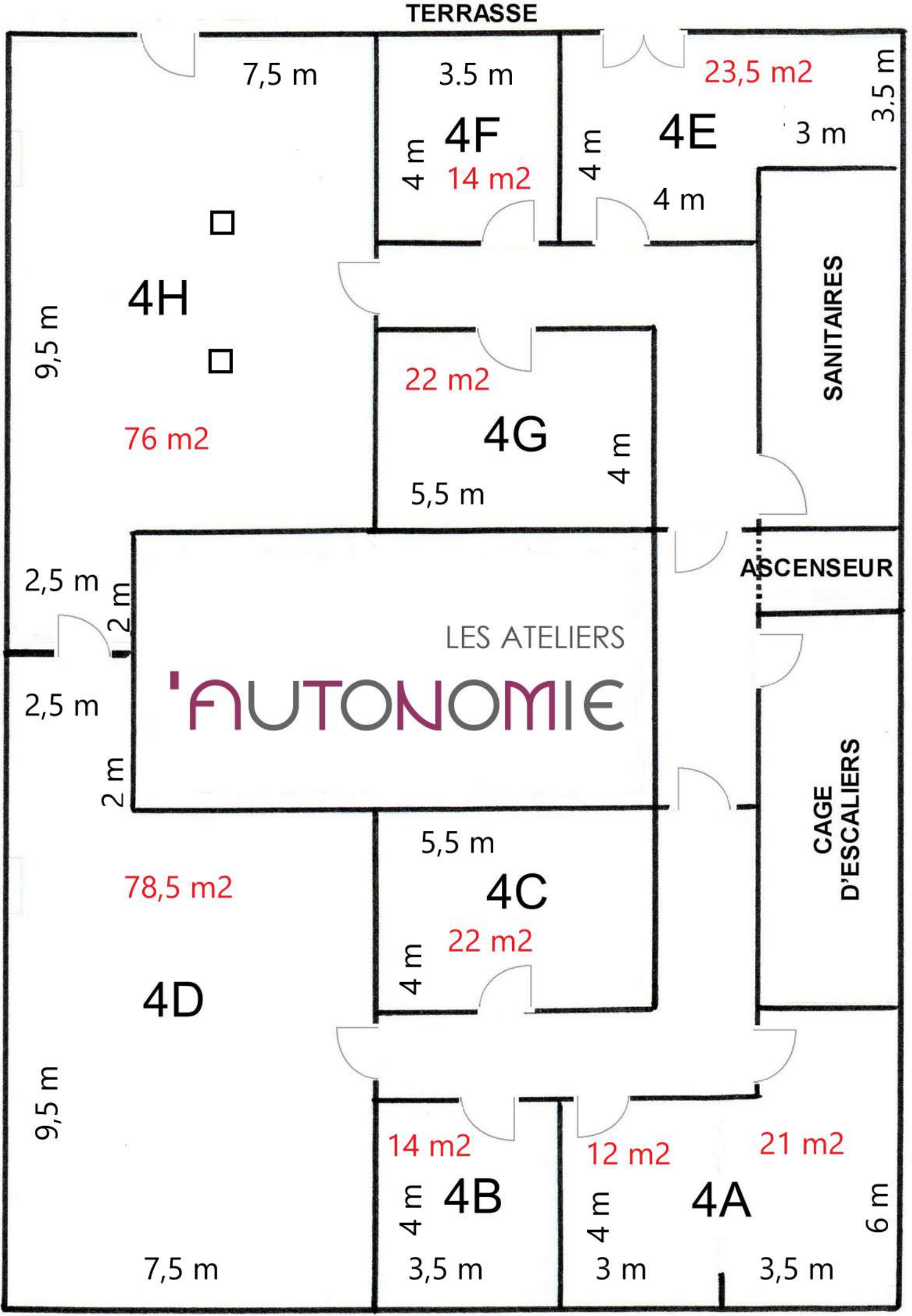
QUATRIEME ETAGE
